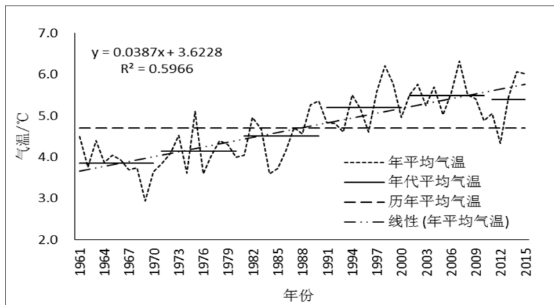
图 1 1961-2015 年草原年平均气温变化
