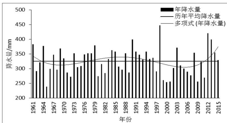
图 2 1961-2015 年草原年降水量变化
