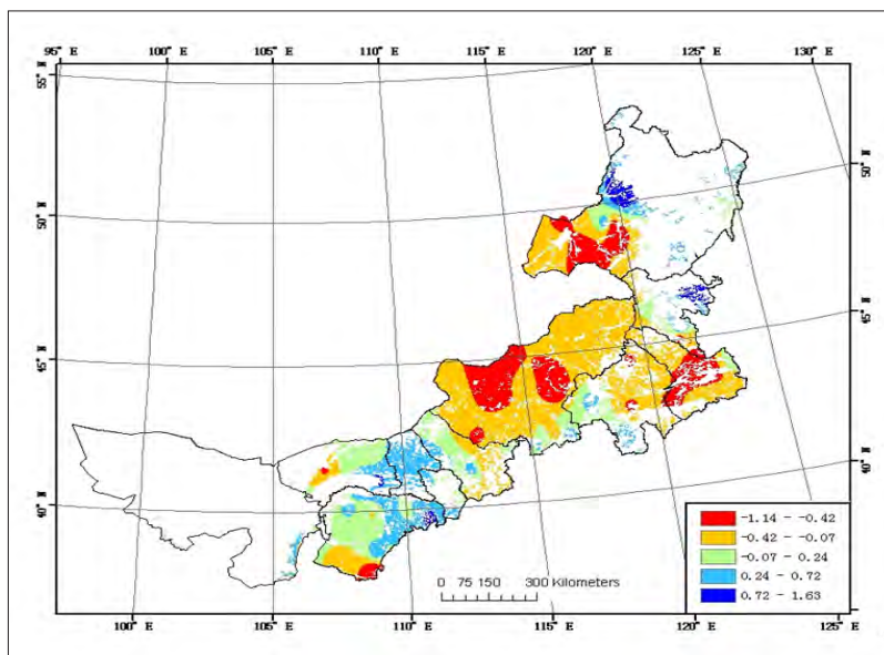
图4 1961-2015年草原年最大地上生物量变化速率空间分布(克/平方米年)
